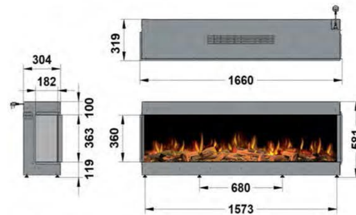
1650 - LEFT CORNER
